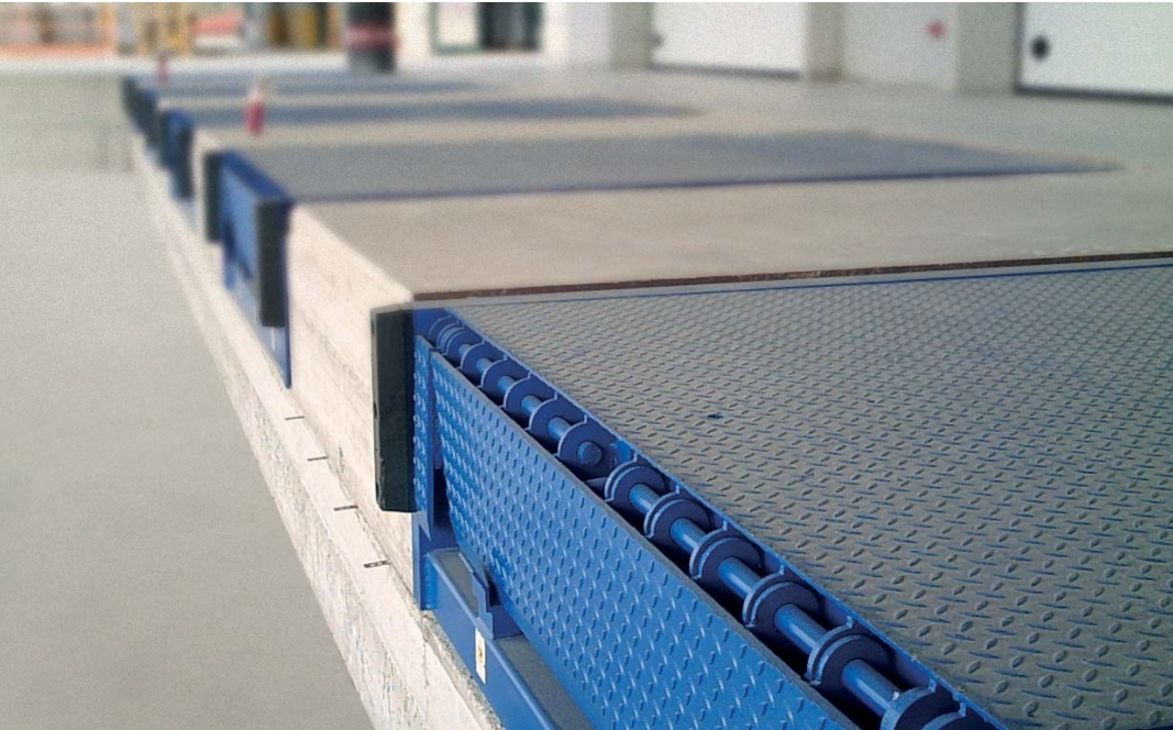
Pedana con Spondina Rotante Dock Leveller with up turned lip Ladebühne mit umlaufender Klappe
